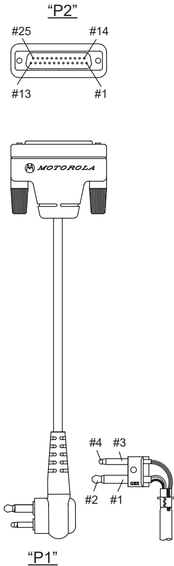
Figura 2: Cabo de Teste Portátil (PMKN4156_ )
