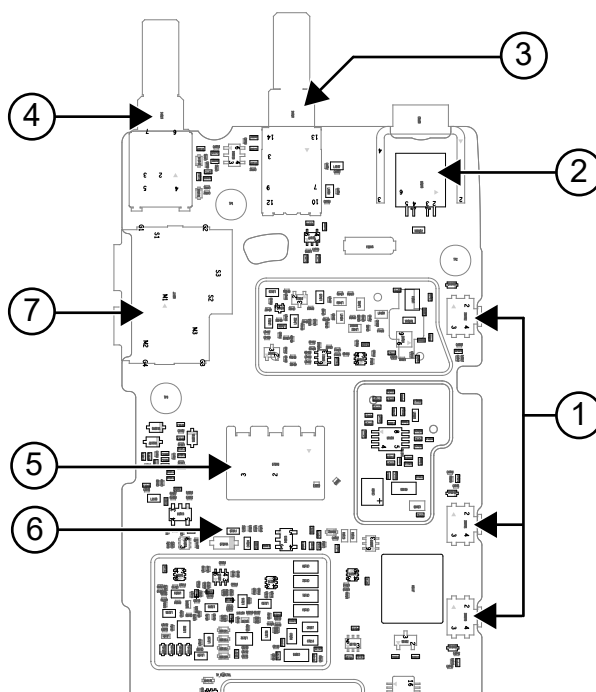
Figure 6 : Partie supérieure de la carte mère pour VHF
