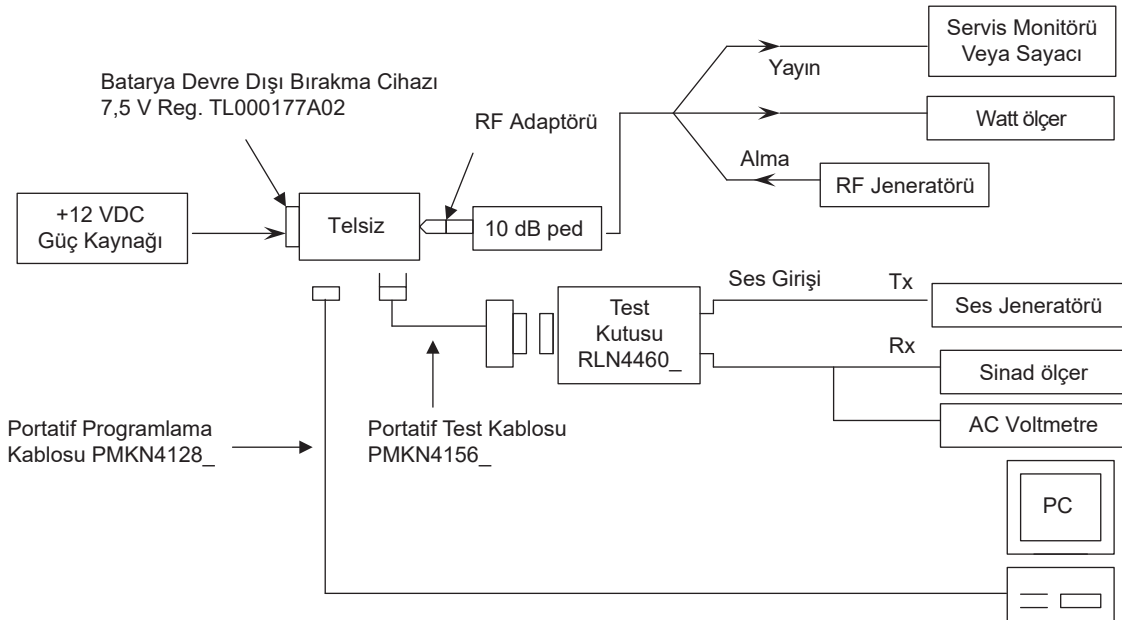
Şekil 4: Telsiz Akordu Ekipmanı Kurulumu
