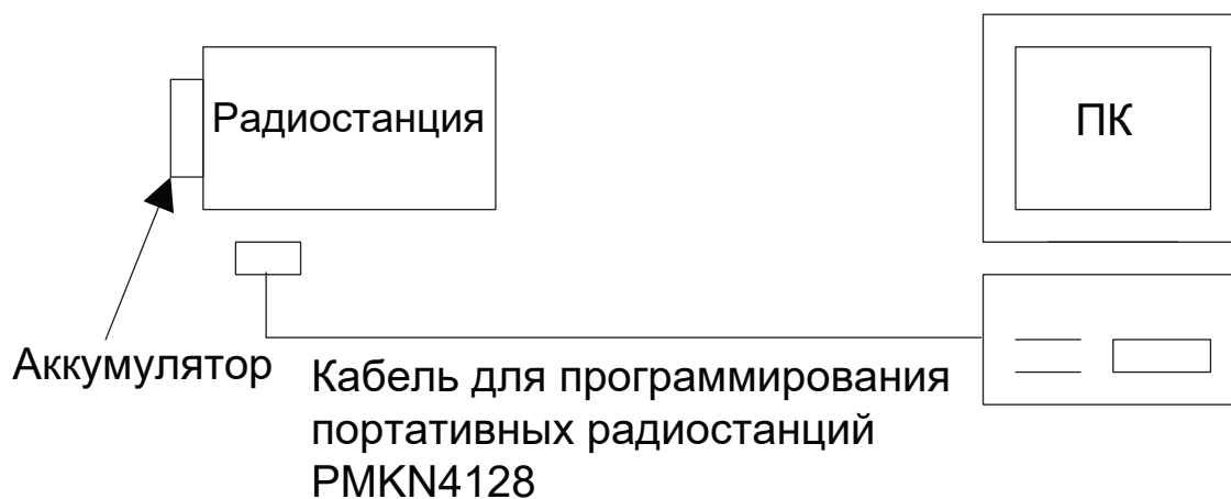
Рис. 3. Конфигурация для программирования с помощью ПО CPS
