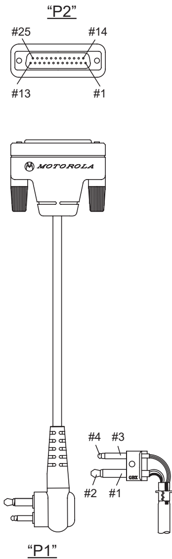
Figura 2: Cable de prueba portátil (PMKN4156_)
