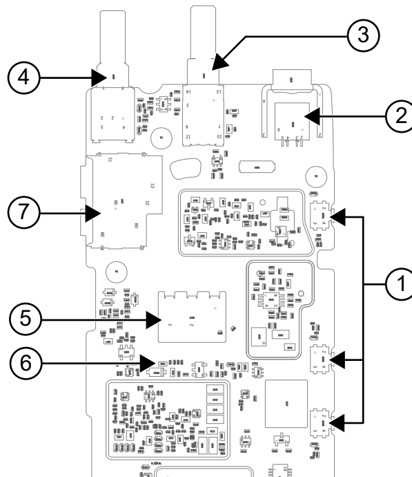
Figura 5: Parte superior de la placa principal para UHF1, UHF2 y la banda de 350 MHz
