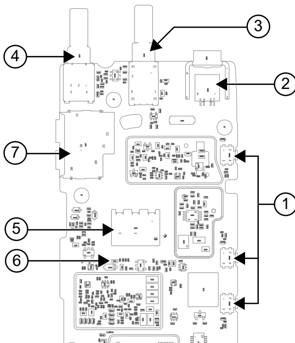
Rysunek 5: Górna strona płyty głównej dla pasm UHF1, UHF2 i 350 MHz
