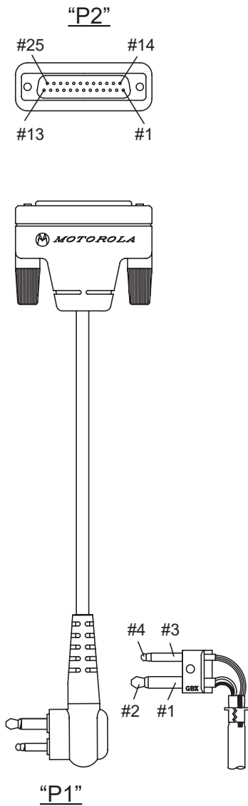
Abbildung 2: Tragbares Testkabel (PMKN4156_)
