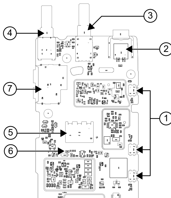
Rysunek 6: Górna strona płyty głównej dla VHF
