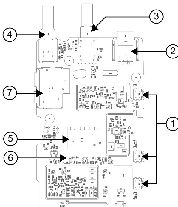
Рис. 5. Верхняя сторона основной платы для диапазона УВЧ1, УВЧ2 и 350 МГц
