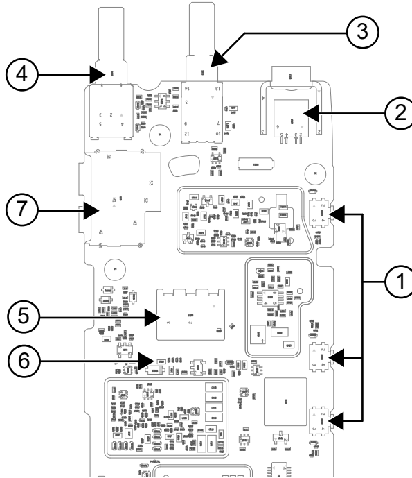
Şekil 5: UHF1, UHF2 ve 350 MHz Bant için Ana Kartın Üst Tarafı
